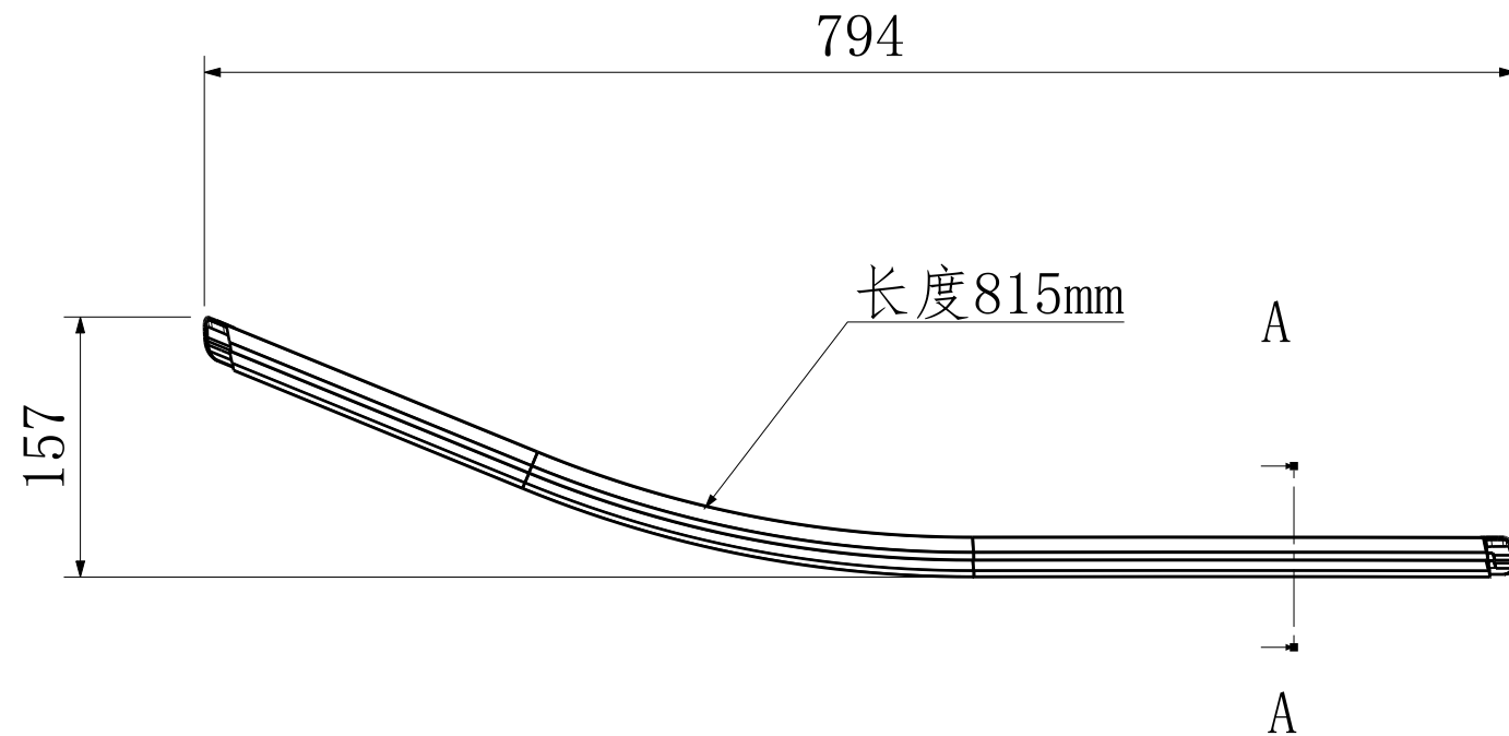
正视图 缩放: 1:5
