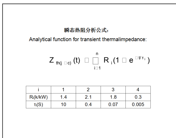
图9. 瞬态热阻抗分析算公式
