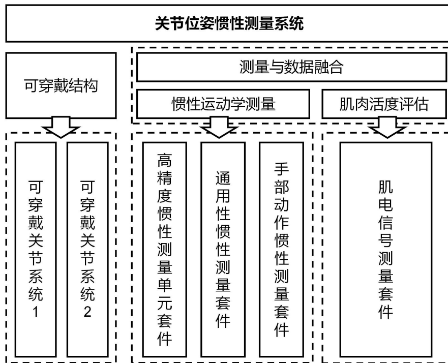
图 1 关节位姿惯性测量系统功能组成示意图
