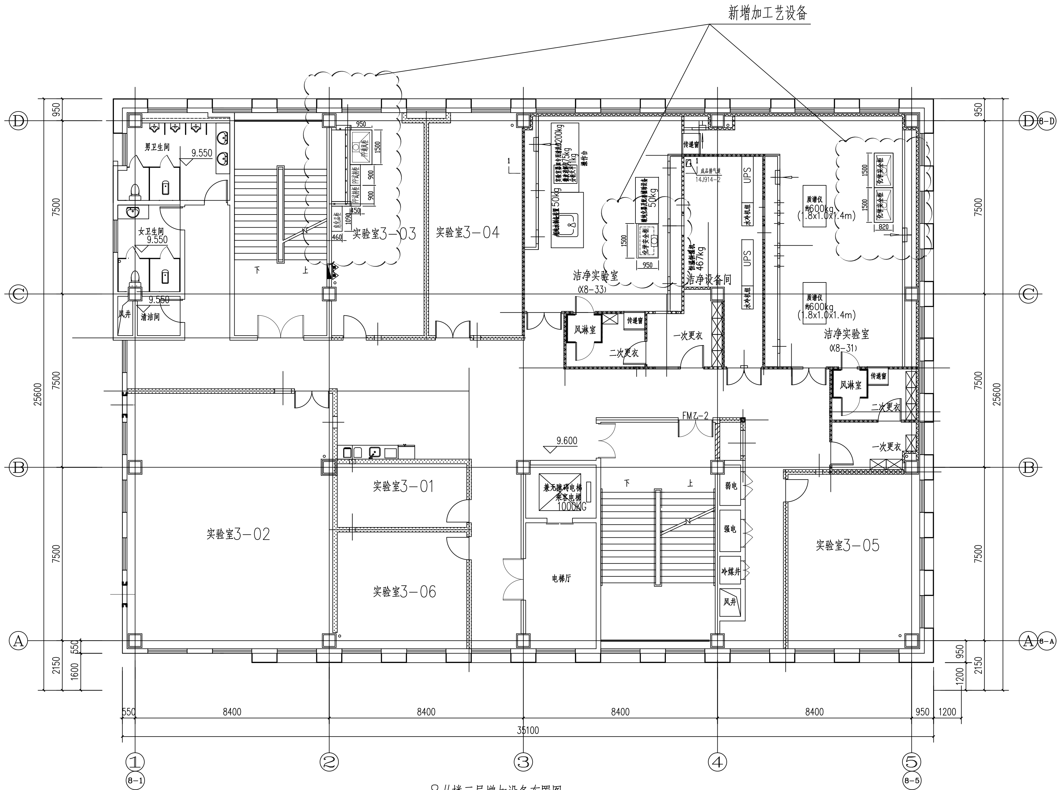
8#楼三层增加设备布置图
