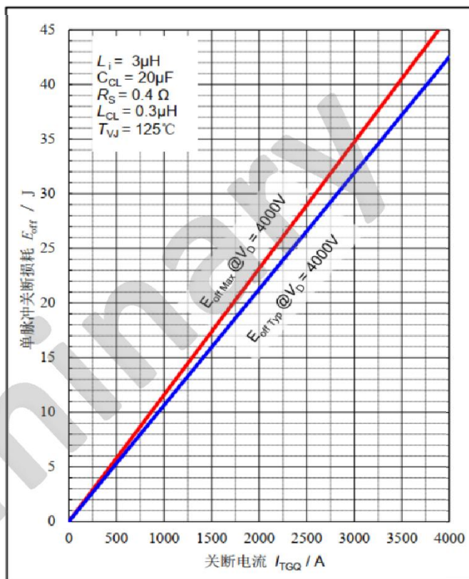
图2. 单脉冲关断能量与关断电流的关系曲线
