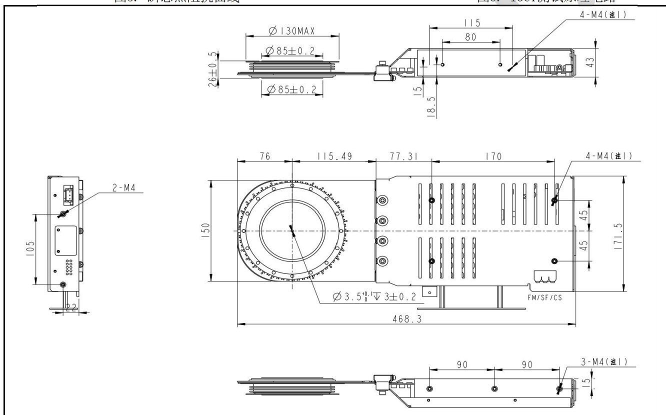
图7. IGCT器件外形图 (单位: mm)
