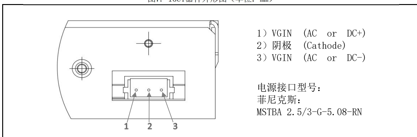
图8. 门极单元电源接口引脚图
